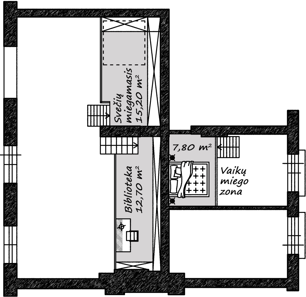
Antresolės - 35,70 m 2
