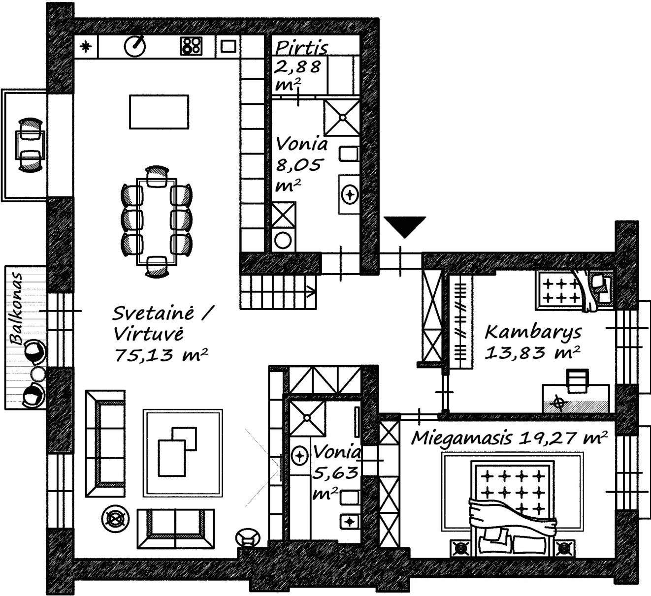
1 lygis - 124,79 m 2
