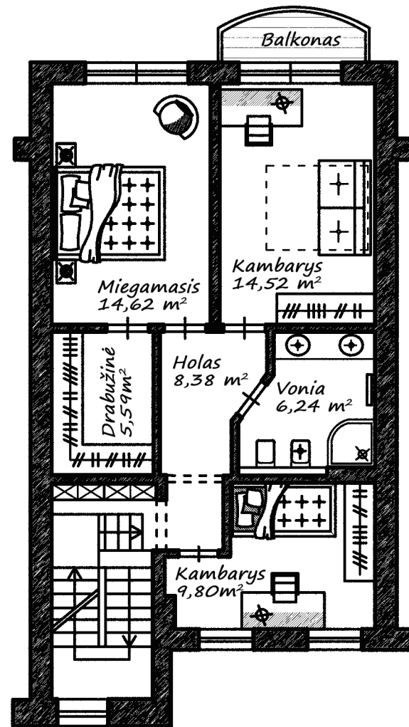
II aukštas 59,15 m 2
